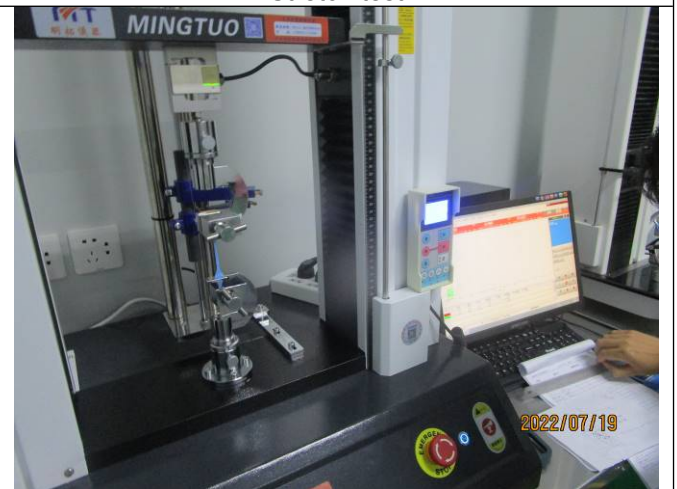
Tensile test
